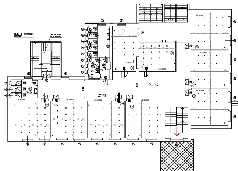
PIANO PRIMO
