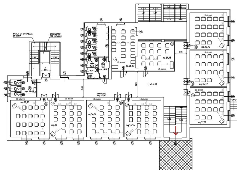
PIANO PRIMO
